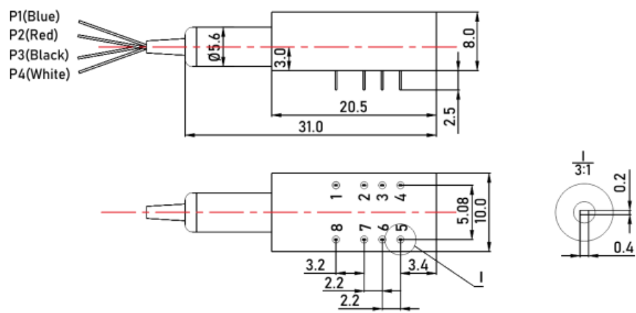
Mini 2×2B 继电器式小型光开关（L20.5×W10×H8.0）
