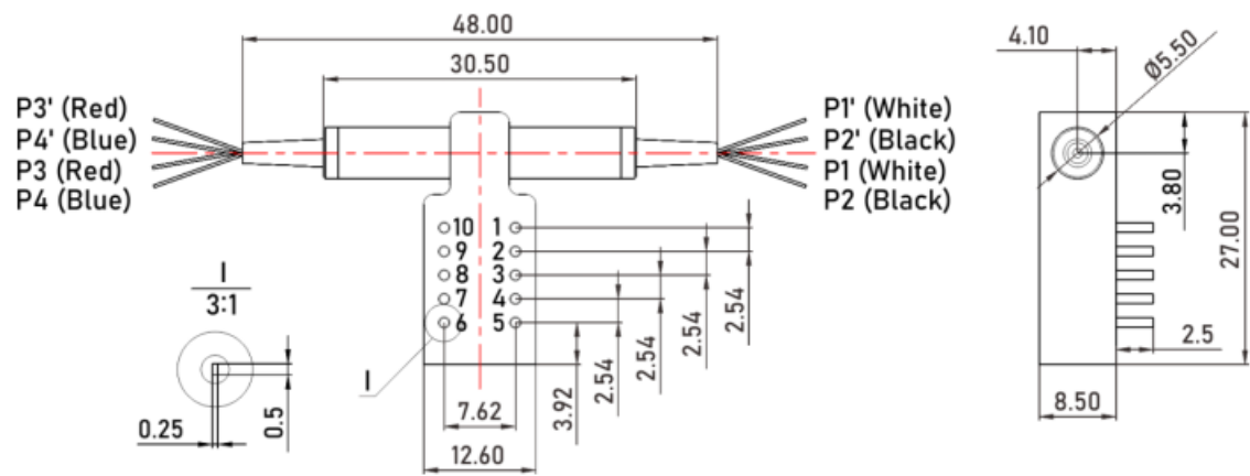
D2×2 PM 继电器式小型光开关（L27×W12.6×H8.5）
