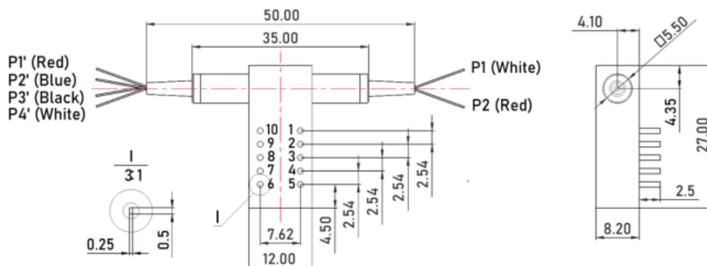
D1×2 PM 继电器式小型光开关 (L27×W12×H8.2)
