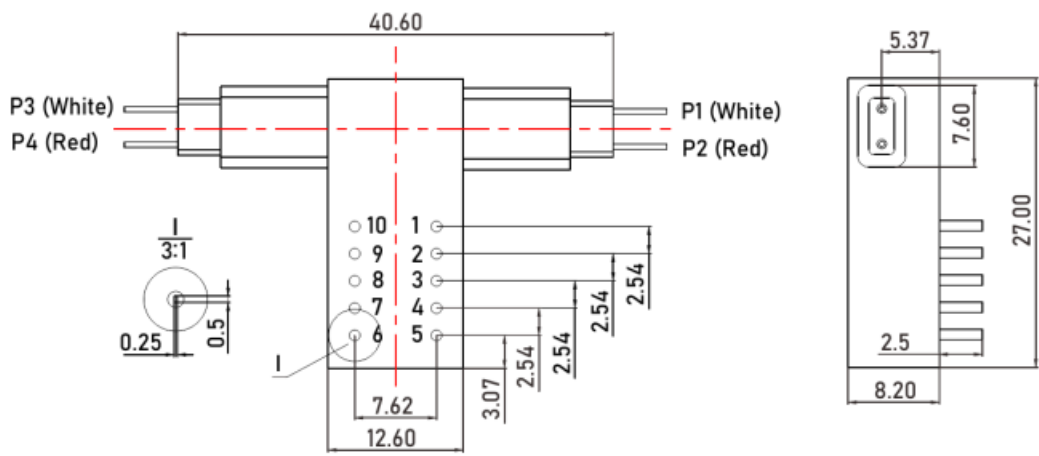
2×2T PM 继电器式小型光开关（L27×W12.6×H8.2）
