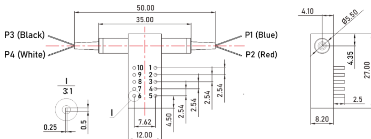
2×2B PM 继电器式小型光开关 (L27×W12×H8.2)
