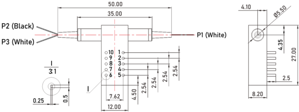
1×2 PM 继电器式小型光开关（L27×W12×H8.2）
