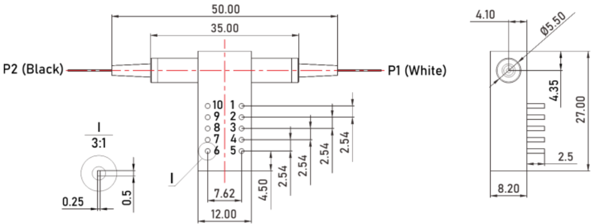
1×1 PM 继电器式小型光开关（L27×W12×H8.2）
