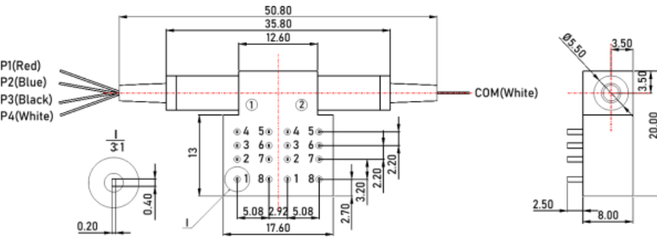
Mini 1×4 继电器式小型光开关（L20×W17.6×H8.0）
