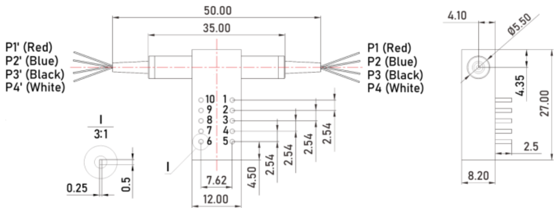
D2×2B 继电器式小型光开关（L27×W12×H8.2）
