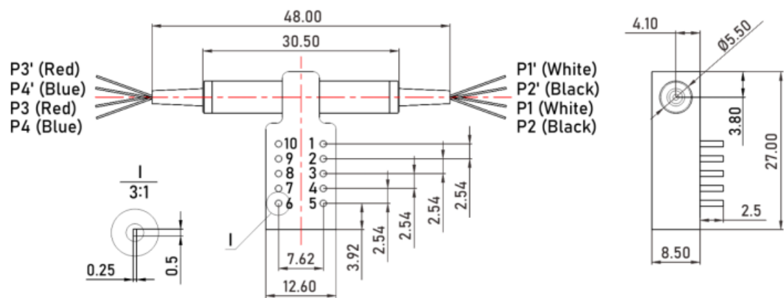
D2×2 继电器式小型光开关（L27×W12.6×H8.5）
