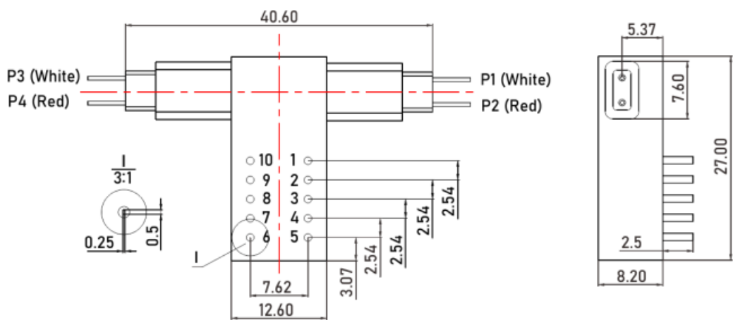
2×2T 继电器式小型光开关（L27×W12.6×H8.2）
