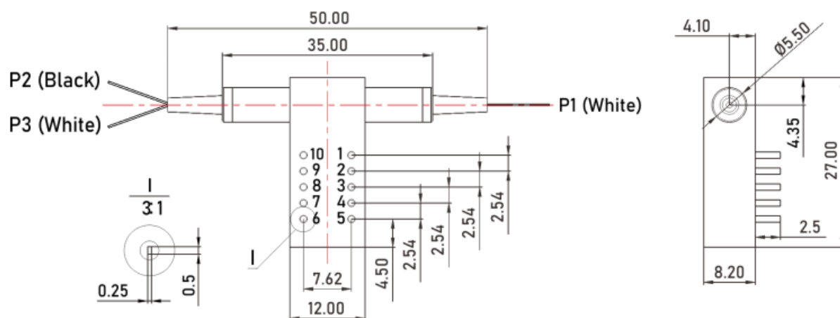
1×2 继电器式小型光开关 (L27×W12×H8.2)
