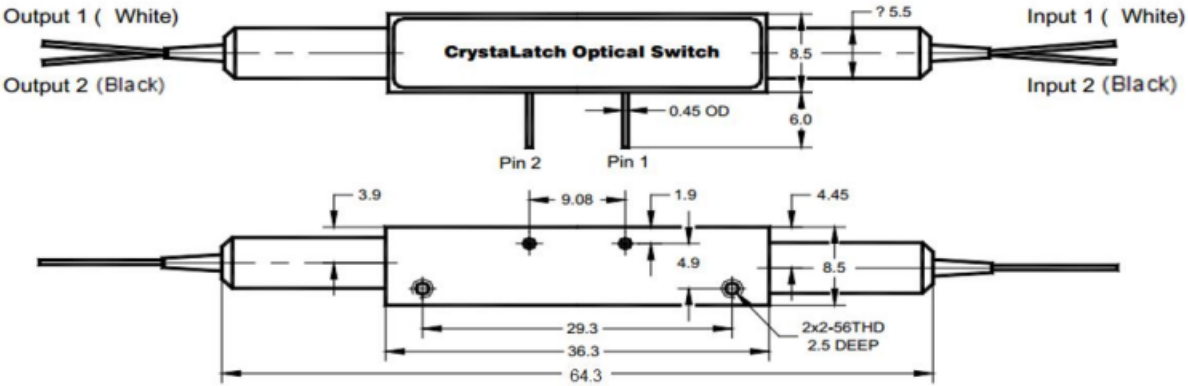
2×2 磁光开关（L64.3×W8.4×H8.4）
