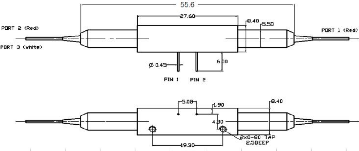
1×2 磁光开关（L55.6×W8.4×H8.4）
